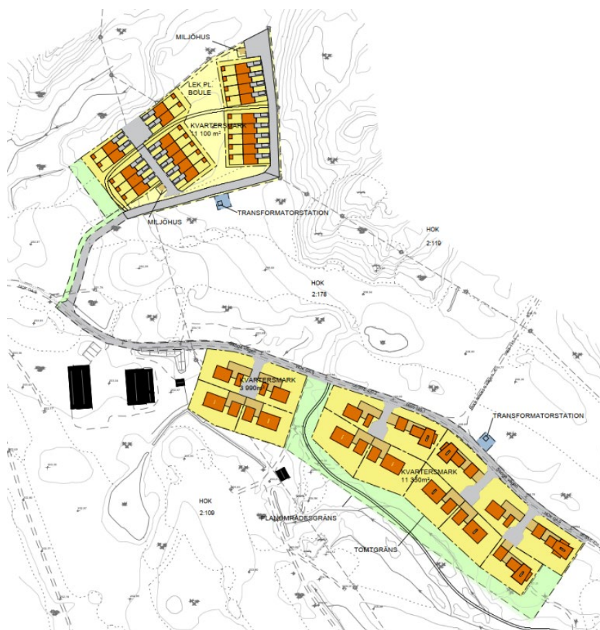
Illustration som visar ett exempel på hur bebyggelsen i planområdet kan utformas, framtaget av bsv arkitekter & ingenjörer ab (2023).
