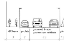
Typsektion och plan Skala 1:200 i A3
