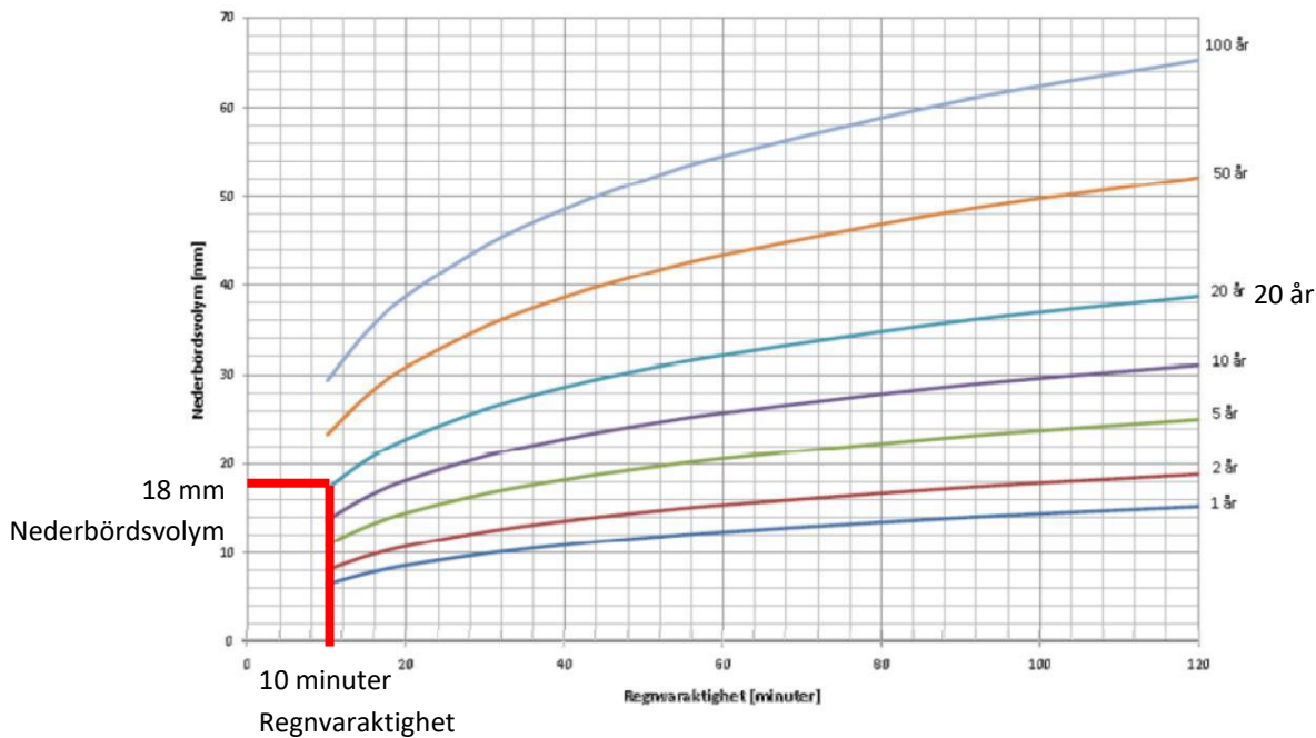
Figur 19. Nederbörsvolym som funktion av regnvaraktighet och återkomsttid från rekommendation svenskt vatten P110.
