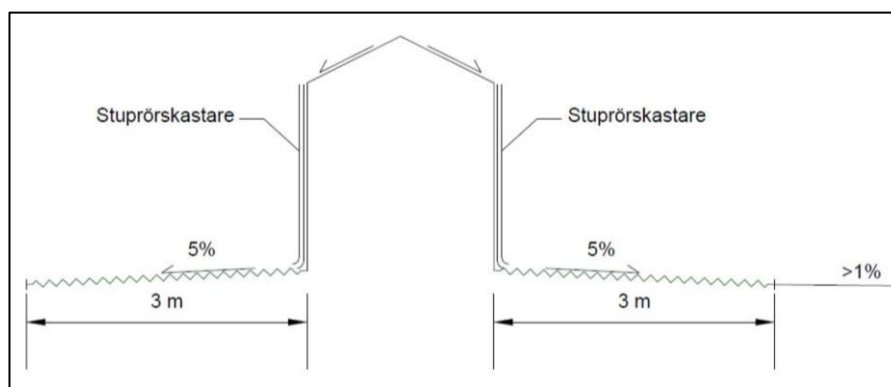
Figur 18. Principskiss över rekommenderande lutningar från byggnader för att undvika att yt- och dagvattnet ställer sig intill huskropp (Bild: Sweco).
