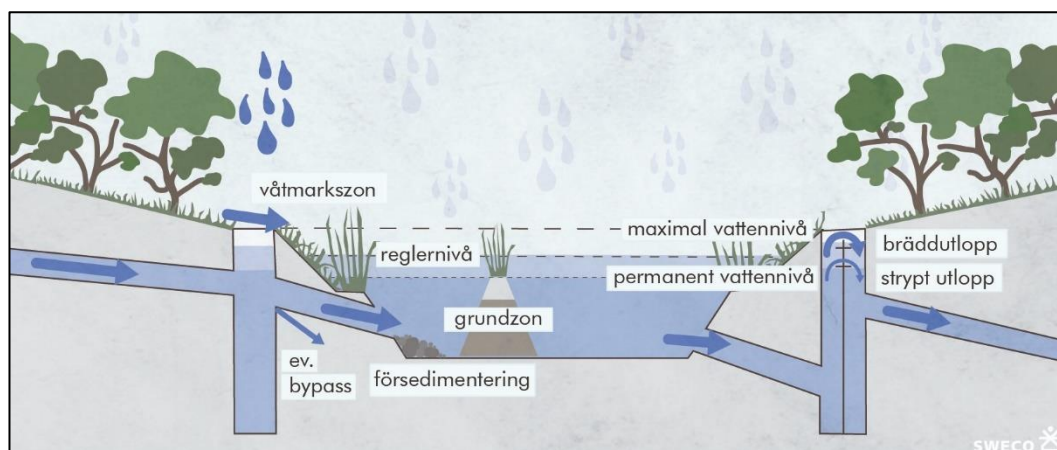
Figur 12. Principskiss över en dagvattendamm (Bild: Sweco).
