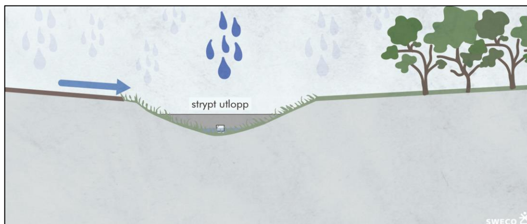
Figur 15. Schematisk bild över ett svackdike (Sweco).
