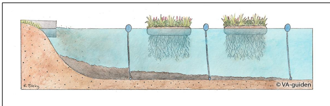
Figur 14. Principskiss på flytande våtmark (Källa: VA-guiden).
