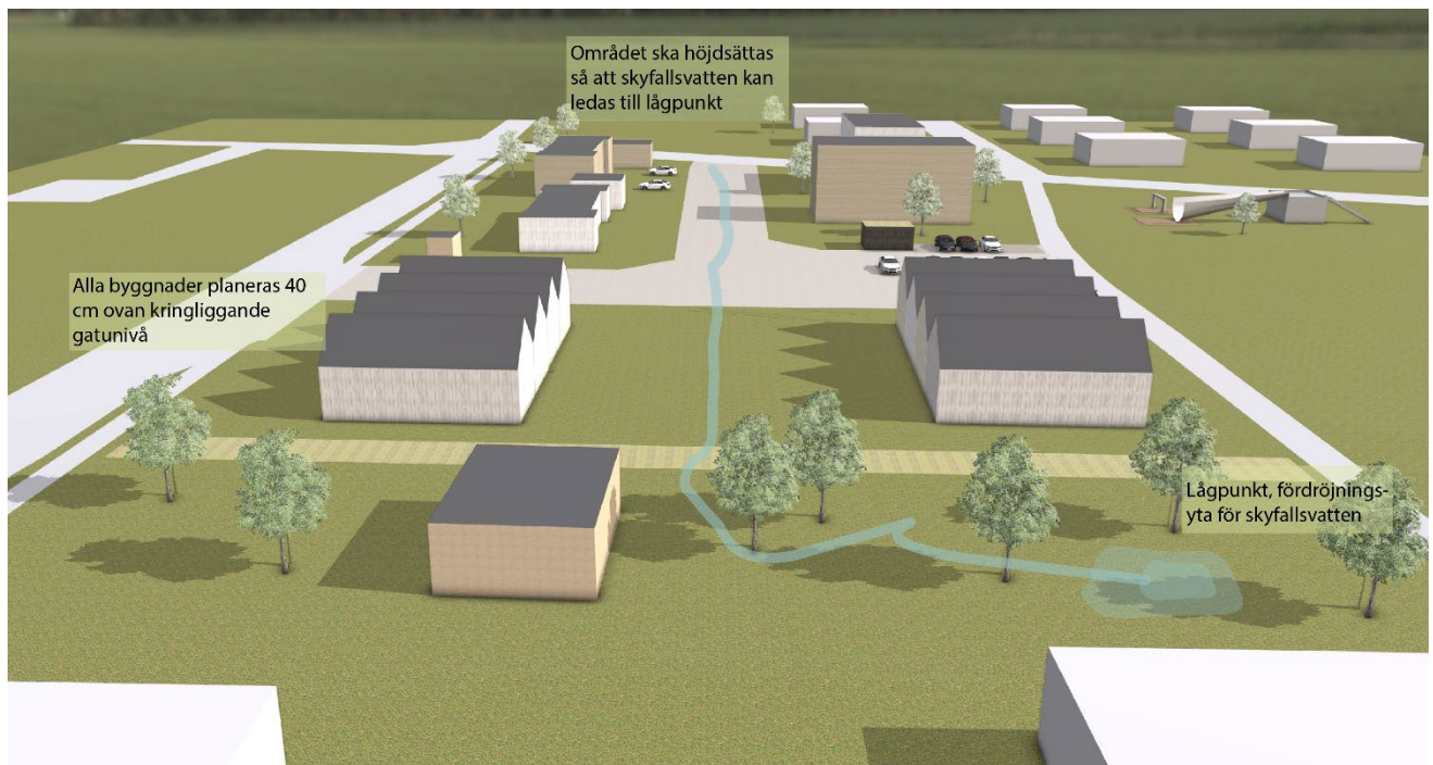
Figur 15. Förslag på ytvattenrening och avledning mot planområdets naturliga lågpunkt i sydöst.
