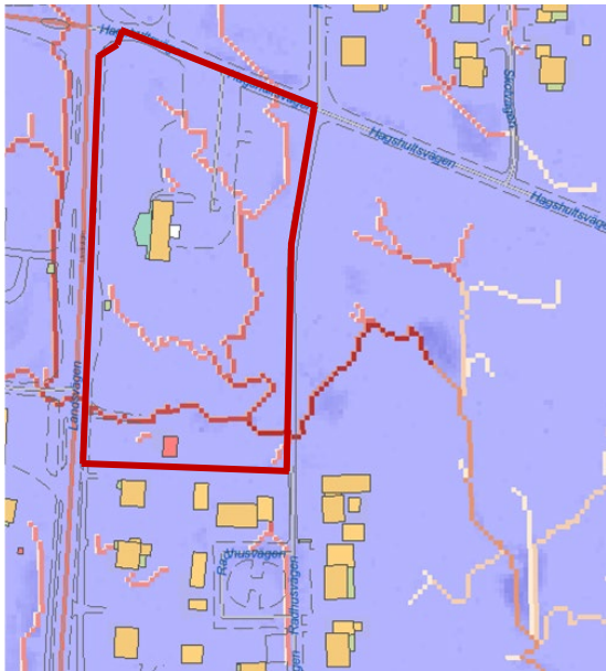
Figur 13. Skyfallskartering från Jönköpings läns Länsstyrelse 2022. Planområdet är markerat med röd linje.
