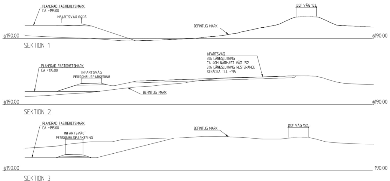
Figur 15 CAD-ritning (förslagsskiss), huvudsektioner.
