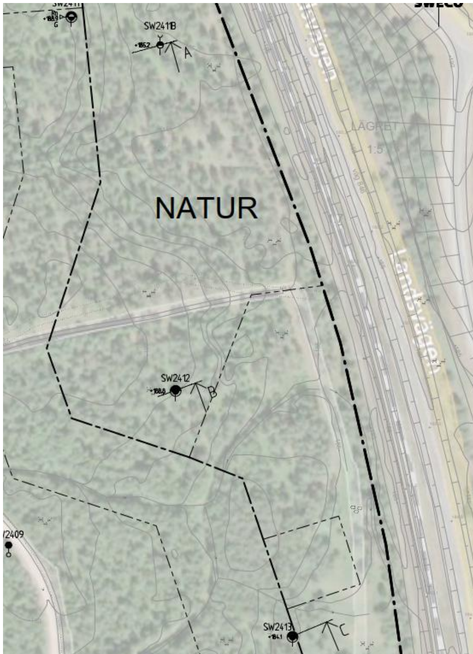
Figur 4. Utklipp ur planritning 30075226-G1, geoteknisk undersökning Sweco 2024. Observera att egenskapsgränsen för naturmarksområdet har ändrats.
