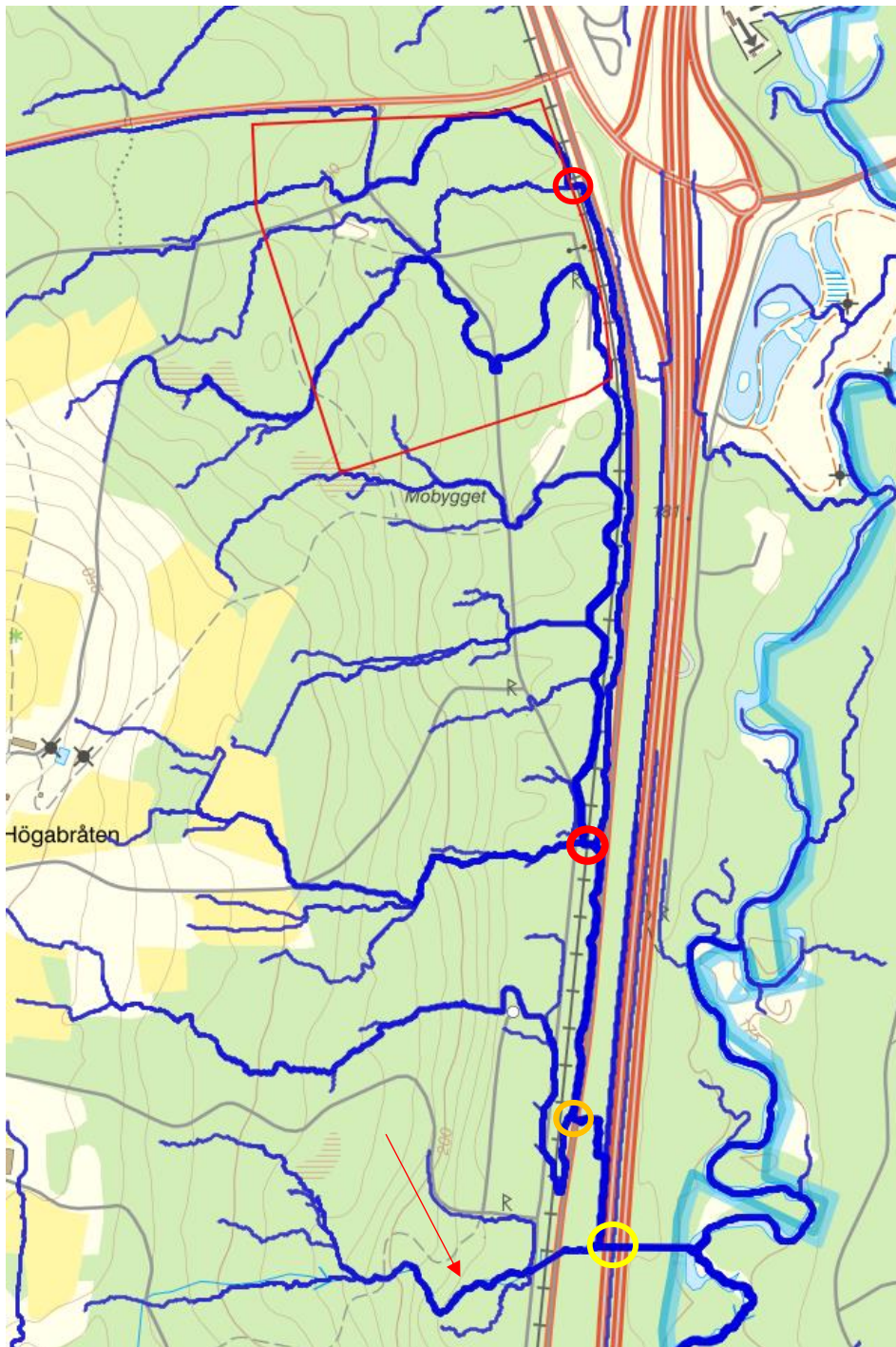
Figur 11. Flödesvägar då samtliga lågpunkter inom området är fyllda till max (se vidare metod i avsnitt 8). Röda cirklar visar inmätta trummor under järnvägen (norra – plåt 600 mm, södra - plast 600 mm), orange cirkel visar placering av trumma under landsvägen enligt trafikverkets databas (500mm) och gul cirkel visar kulvert under E4 enligt trafikverkets databas (800mm). Röd pil pekar på det oklassade vattendrag som leds under E4 och ansluter till Lagan. Generell flödesriktning är åt sydost.
