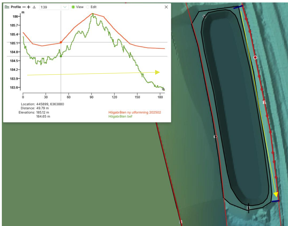
Figur 32. Inlagd nivå på serviceväg intill fördröjningsytan – endast grov skiss för att se till att vatten inte stiger mot järnvägen. Profilen visar riktning från norr till söder.
