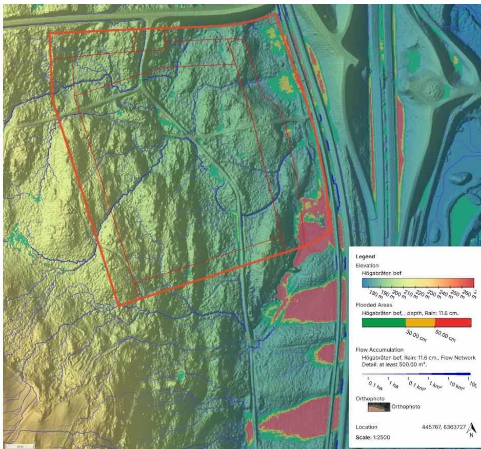
Figur 30. Uppskattning av översvämmade ytor (graderat från grönt till rött efter uppskattat vattendjup) samt flödesvägar som har uppströms avrinningsområden >500 m 2 (blå linjer) vid en regnbelastning på 116 mm. Modellen baseras på befintlig situation med höjddata från nationella höjddatabasen.
