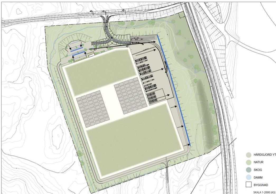
Figur 22. Principskiss över hur makadamdiken eller växtbäddar (blå linjer) kan placeras för att samla upp ytvavrinnande vatten från hårdgjorda ytor. Svarta pilar visar marklutning. Utkast på illustration, Kaminsky, 2025-03-03.
