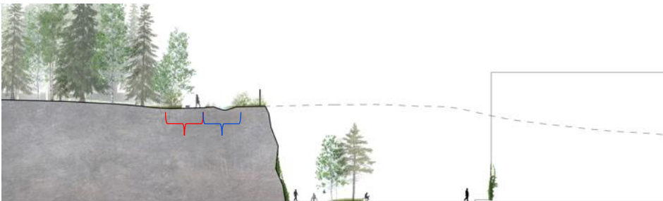
Figur 27. Sektion över den västra delen av planområdet med avskärande dike (blå klammer) ovan slänt. Väg ovan slänten markerad med röd klammer.
