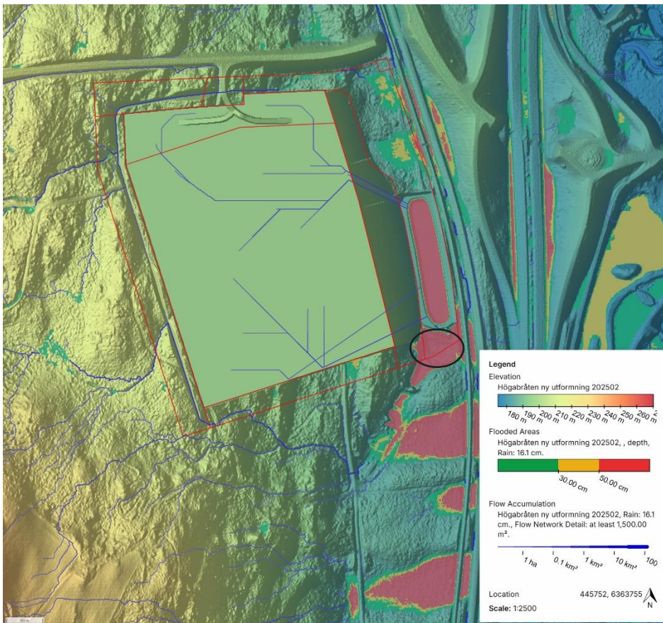
Figur 31. Uppskattning av översvämmade ytor (graderat från grönt till rött efter uppskattat vattendjup) samt flödesvägar som har uppströms avrinningsområden >500 m 2 (blå linjer) vid en regnbelastning på 116 mm. Modellen baseras på en uppskattning av höjder efter exploatering där ytan som kommer bebyggas är lagd på +195,5 m ö.h samt slänt i den östra och västra delen av ytan. Höjderna är korrigerade med avskärande åtgärder för naturmarksavrinning i väst samt fördröjningsyta i öst. Del av serviceväg intill fördröjningsytan är inlagd på en miniminivå på +184,8 som lutar mot dammen. I norr är den planerade infarten inlagd enligt preliminärt projekterade höjder med trumma under vägen. Naturlig lågpunkt som bör bevaras markerad med svart cirkel.
