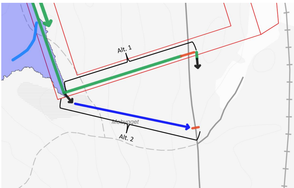
Figur 28. Alternativ för hantering av naturmarksflöden som leds söderut. Grön linje illustrerar dikessträcka, gröna pilar flödesriktning och svarta pilar där vatten släpps i naturmark, röda linjer förslag på placering av trummor och blå linjer naturliga befintliga dikessträckor. Mörkblå pil illustrerar var vatten kommer rinna genom naturmark mot lågpunkt intill väg i alternativ 2.
