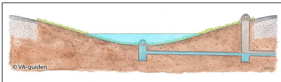
Figur 21. En vattenfylld fördröjningsyta med ett ströpt utlopp i botten (i detta fall på 45 l/s) och ett bräddavlopp vid ytans krön där vatten kan avbördas med högre kapacitet om vatten stiger ända upp till ytans krön. Bild från VA-guiden, 2024–08.
