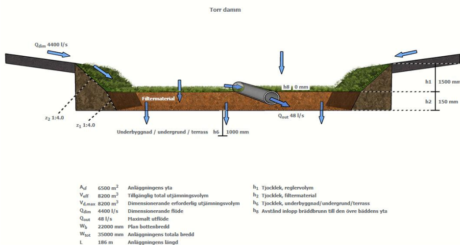
Figur 18. Indata och dimensioner på anläggning, urklipp från beräkning i Stormtac Web 2025-02-25.
