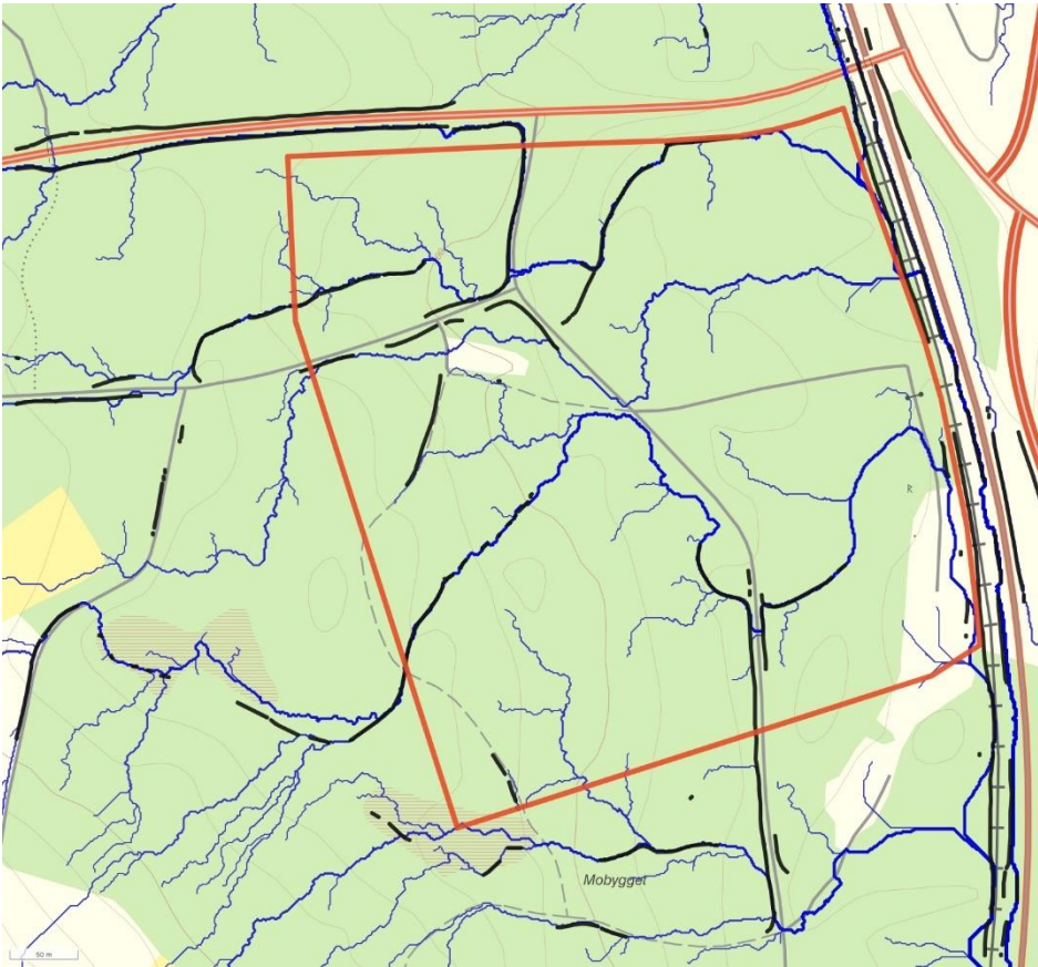
Figur 10. Troliga skogsdiken inom området markerade med svarta linjer. Rinnvägar generade utifrån befintliga marknivåer (depression free flow). Detaljplanområdets gräns är markerat med röd linje. Verktöget baseras på nationella höjddata - Markhöjdmodell, grid 1+ (2023-07-24). Källa: Lantmäteriet hämtat från SCALGO Live (2025).
