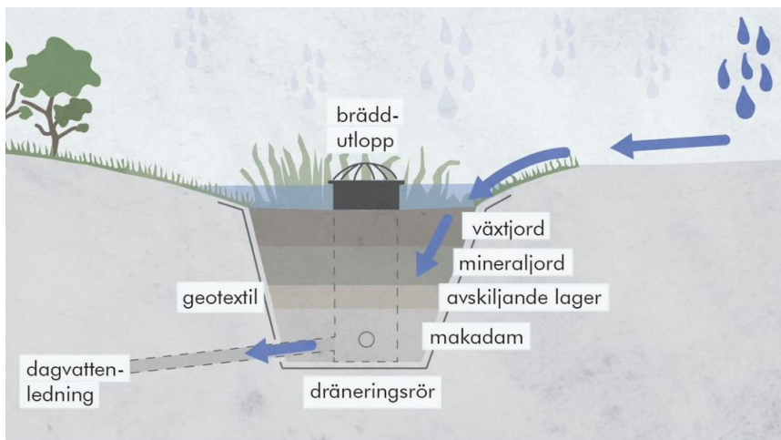
Figur 25. Principskiss för nedsänkt växtbädd med fördröjning ovanpå bädden. Illustration: Sweco.
