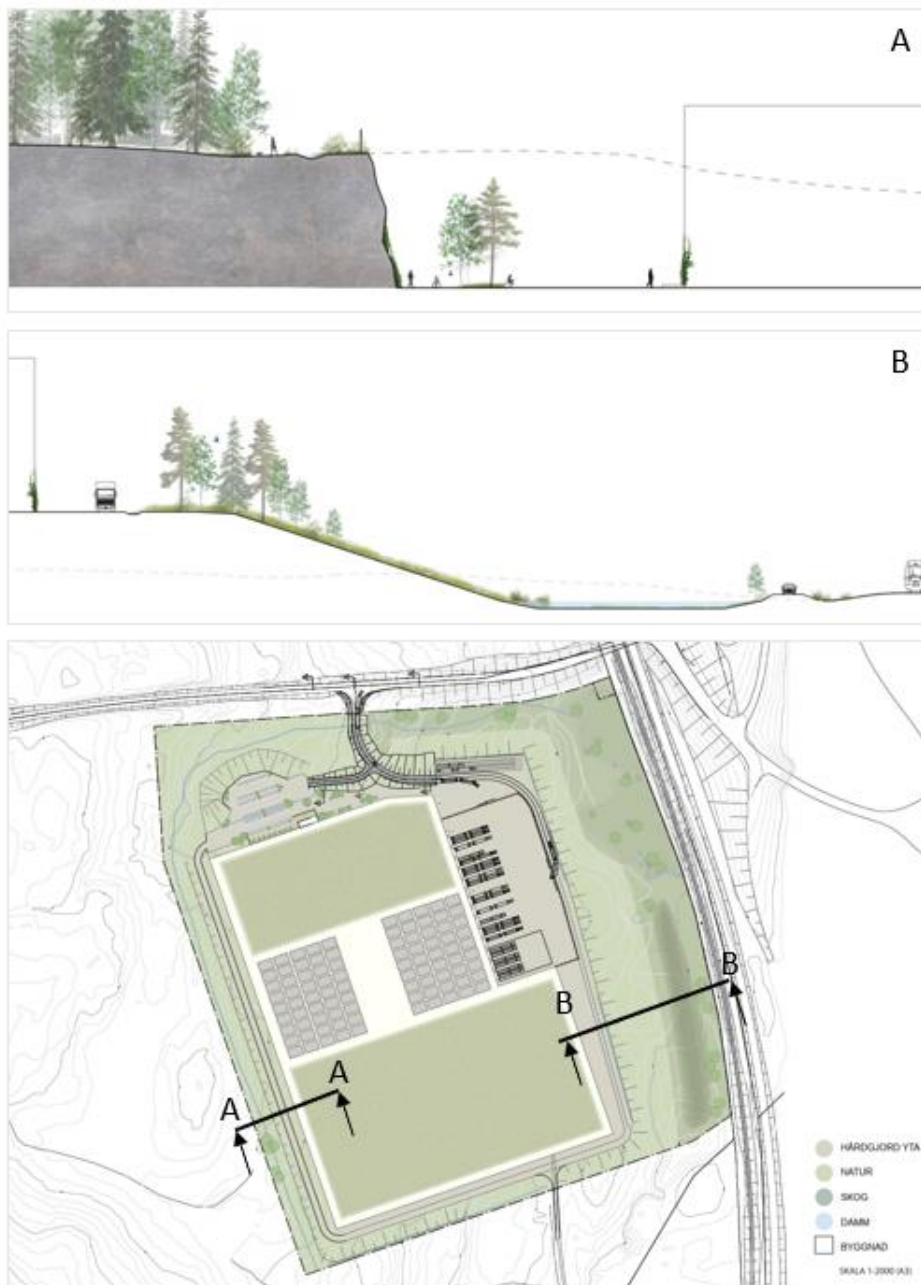
Figur 13. Principskiss över sektion A och B. Urklipp ur arbetsmaterial av gestaltning och sektioner av Kaminsky och Mareld arkitekter, 2025-03-06.
