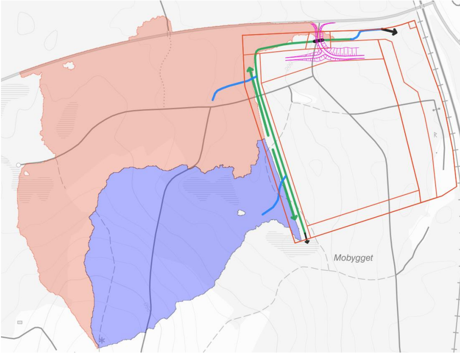
Figur 26. Principskiss över avledning av naturmarksflöden förbi planområdets bebyggda delar. Blått avrinningsområde leds åt söder och rött åt norr. Grön linje illustrerar dikessträcka, gröna pilar flödesriktning och svarta pilar där vatten släpps i naturmark, svart linje visar förslag på placering av trumma under ny infart och blå linjer avslutande naturliga befintliga dikessträckor. Infartens preliminära placering och slänt visas med rosa linje.
