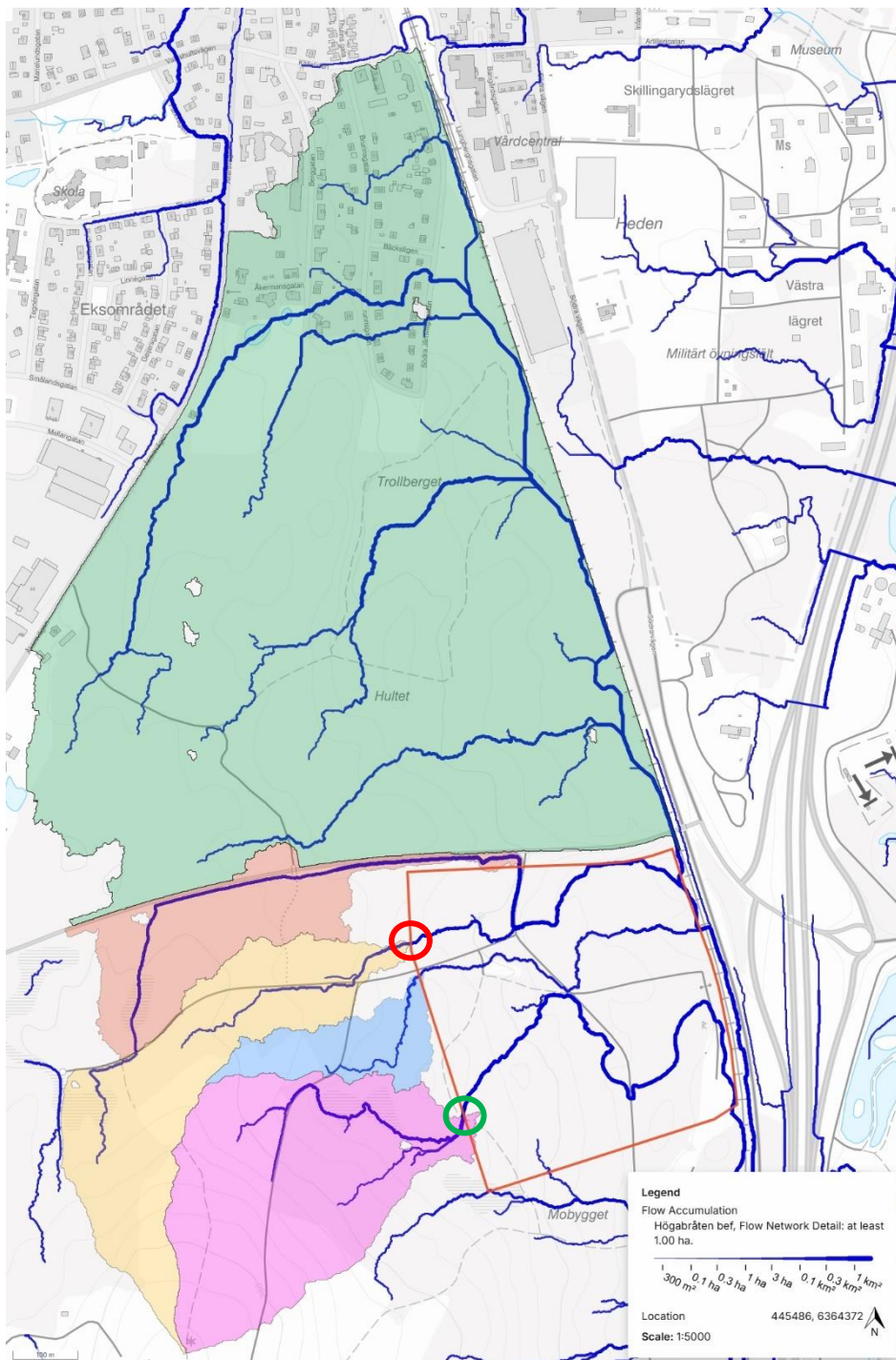
Figur 7. Maximal utbredning av stora avrinningsområden uppströms planområdet som avrinner mot planområdet enligt höjdanalys. Avrinningsområden visas i olika färger och större ytliga flödesvägar visas som blå linjer. Dike i norr inringat med röd cirkel och dike i söder inringat med grön cirkel. Plangräns visas som röd linje.
