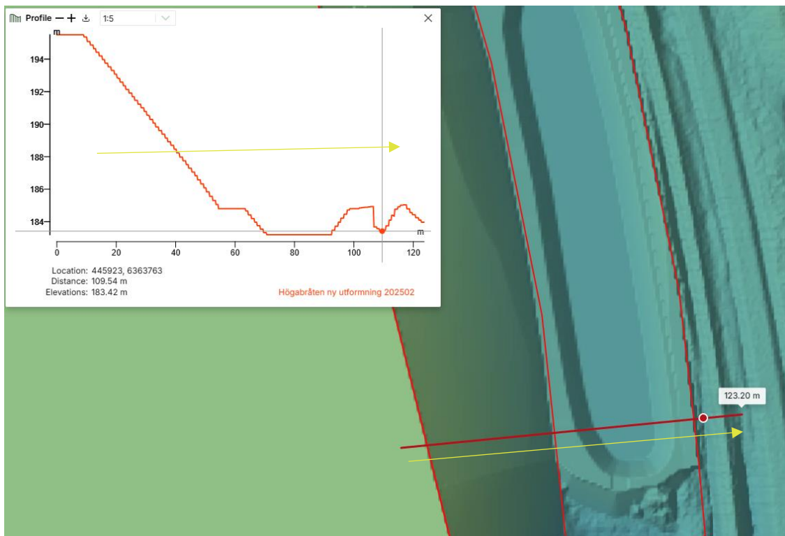
Figur 33. Grov sektion från den byggbara ytan på +195,5 till järnvägen. Järnvägsdiket är markerat med röd punkt i sektion. Profilen visar riktning från väst till öst.
