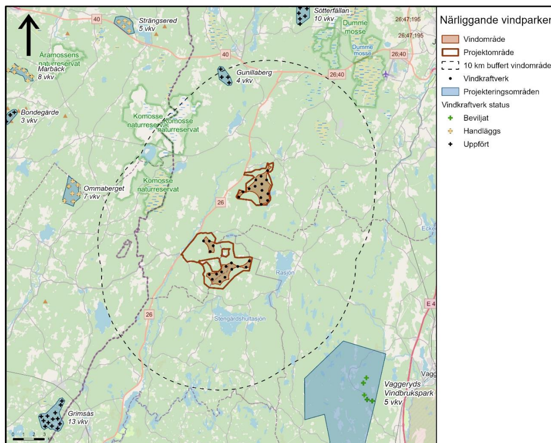
Figur 14: Närliggande vindparker
