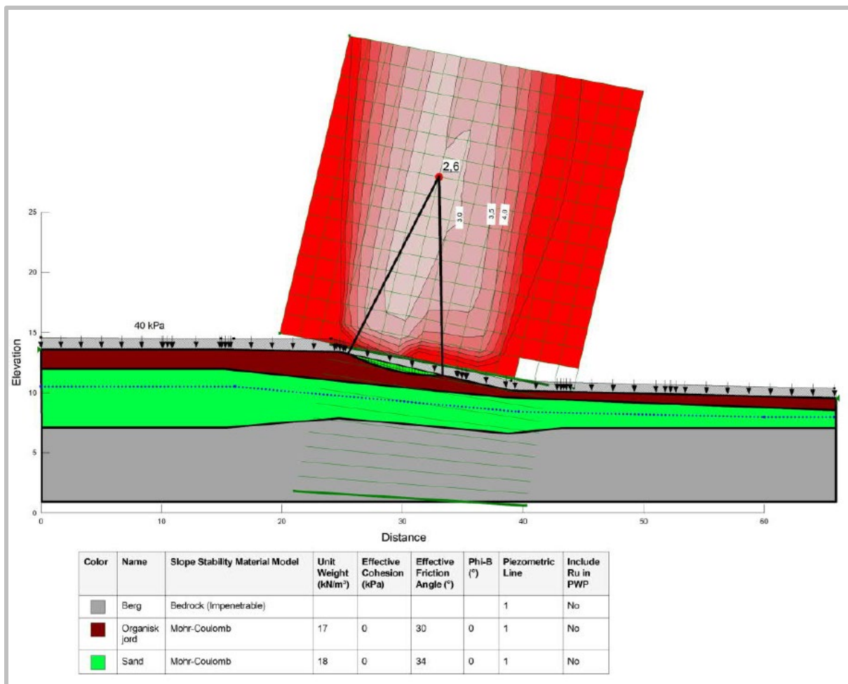
Figur 7: Överslagsmässig stabilitetsberäkning.
