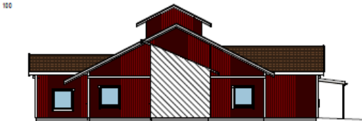
FAÇAD 4 1 : 100
