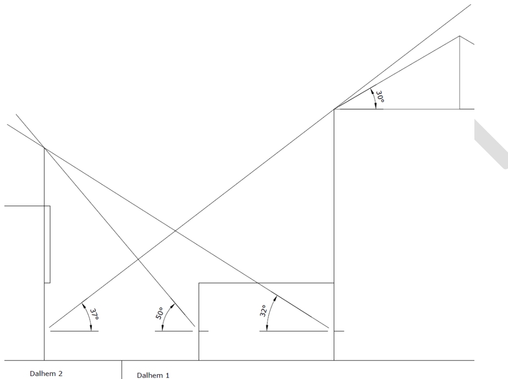
Figur 8: Sektionsskiss Dalhem 1 - Dalhem 2.
