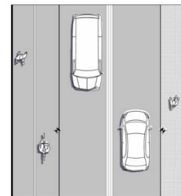
Typsektion och plan Skala 1:200 i A3
