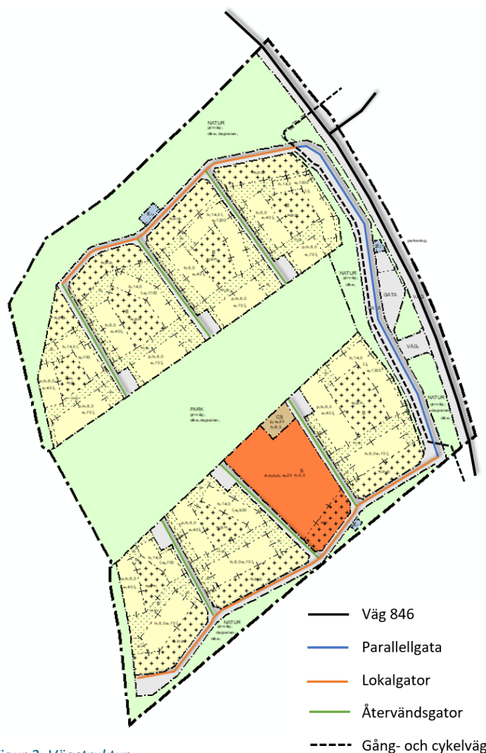
Figur 3: Vägstruktur.
