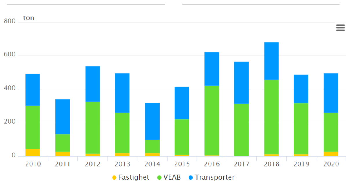
Figur 2. Diagrammet visar mängden direkta fossila koldioxidutsläpp från våra transporter, fastighetsenhetens lokalbestånd samt VEAB:s värmeverk.
