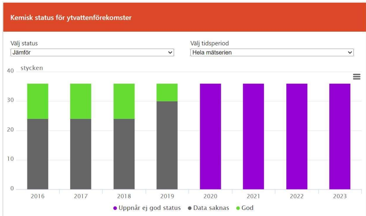
Figur 25. Diagrammet visar den kemiska statusen för ytvattenförekomster i Vaggeryds kommun (Källa VISS).
